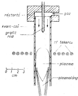
22. ábra. Indukciós plazma-fáklya
