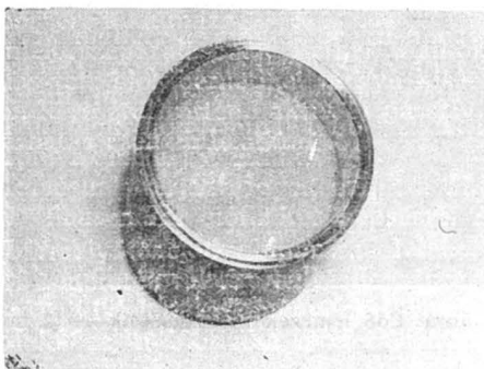
8. ábra. NaI(Tl) kristály foglalásban (átmérője kb. 8 cm)
